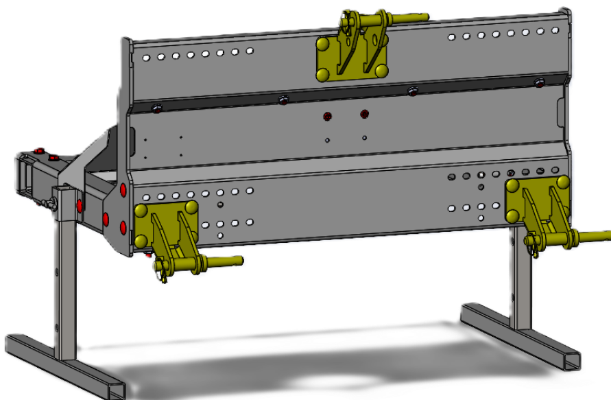
GreenTec FOX-Multiträger mit Halterung für 3-Punkt-Anbau (Kategorie 1 & 2)
