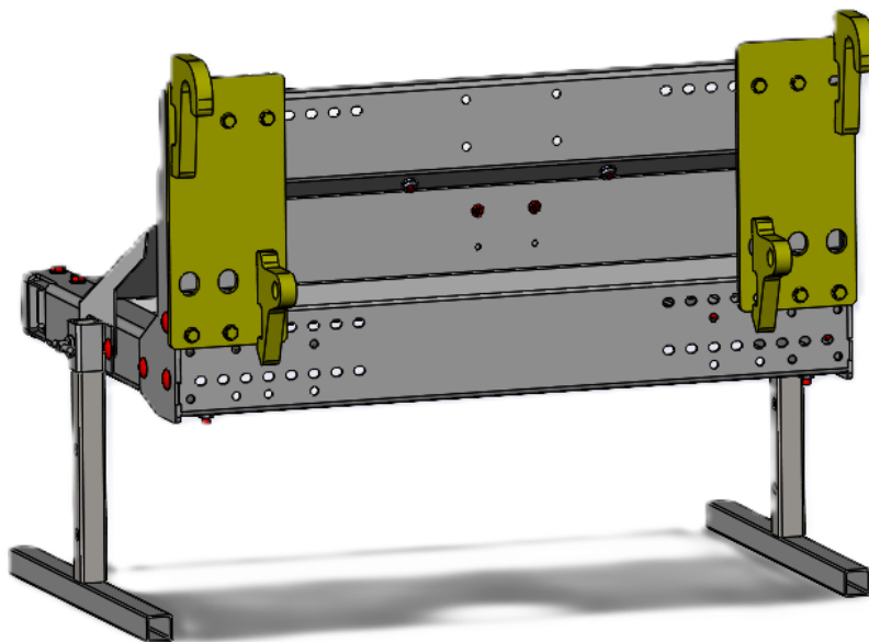
GreenTec FOX-Multiträger mit Euro Hitch Aufnahme
