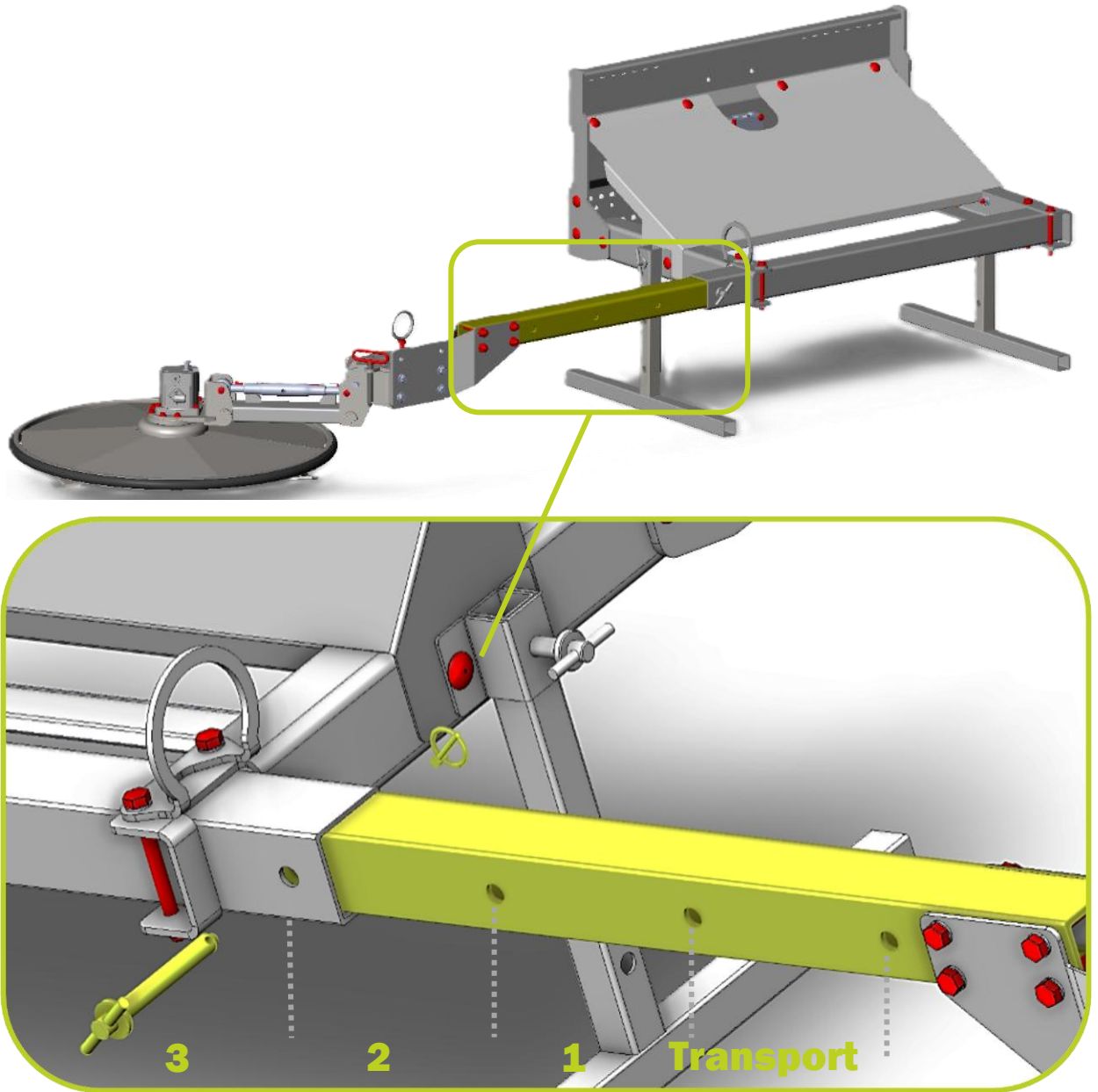
Positionen / Einstellmöglichkeiten der Arbeitspositionen: FOX-Multiträger
