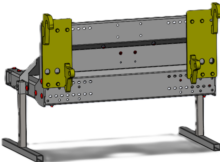
Porte-outil FOX GreenTec avec supports pour chargeur Euro
