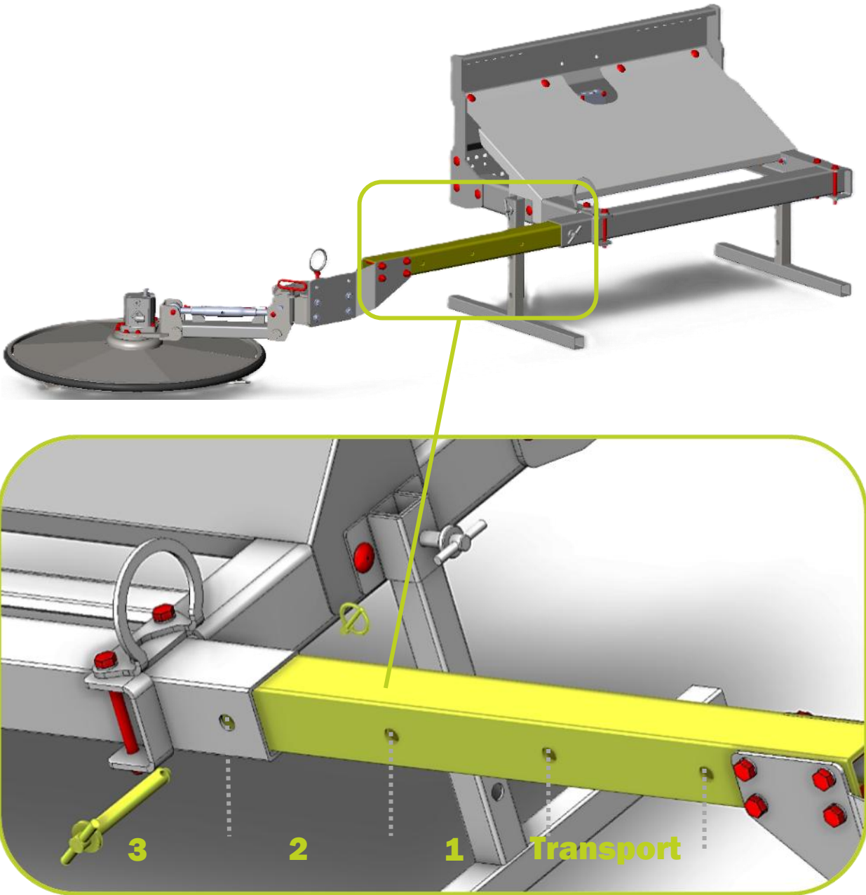
Emplacements/possibilités de réglage des positions de travail : Porte-outil FOX
