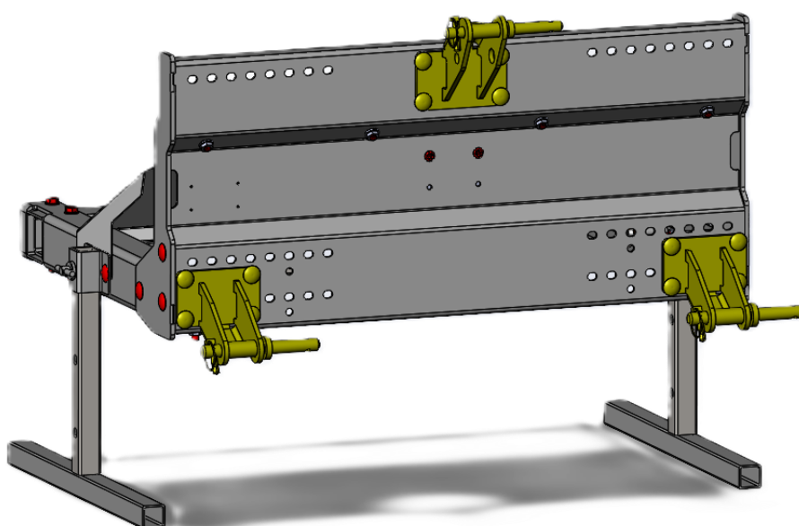
Porte-outil FOX GreenTec avec liaisons d'attelage 3 points (catégorie 1 et 2)
