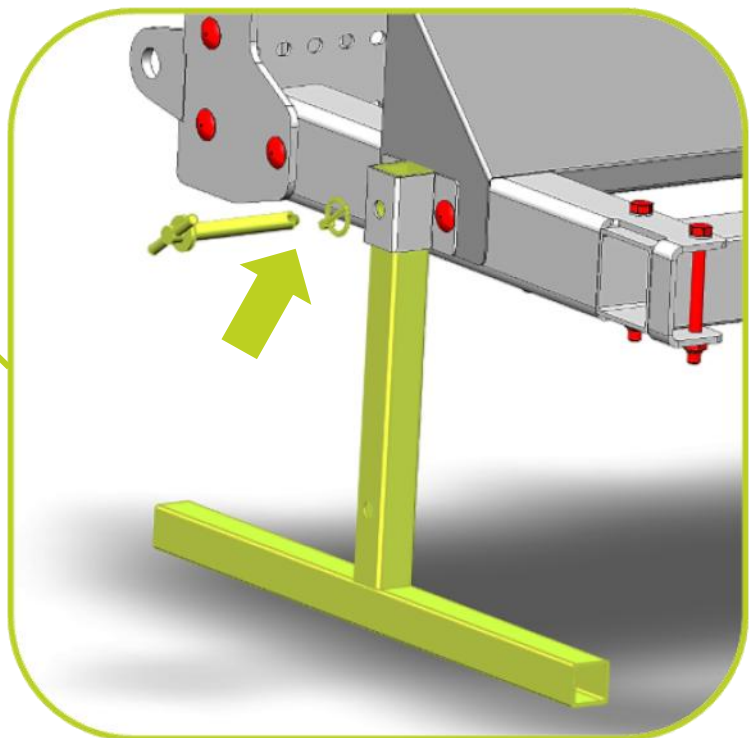
Béquilles avec goupilles de sécurité et goupilles clips : Porte-outil FOX GreenTec
