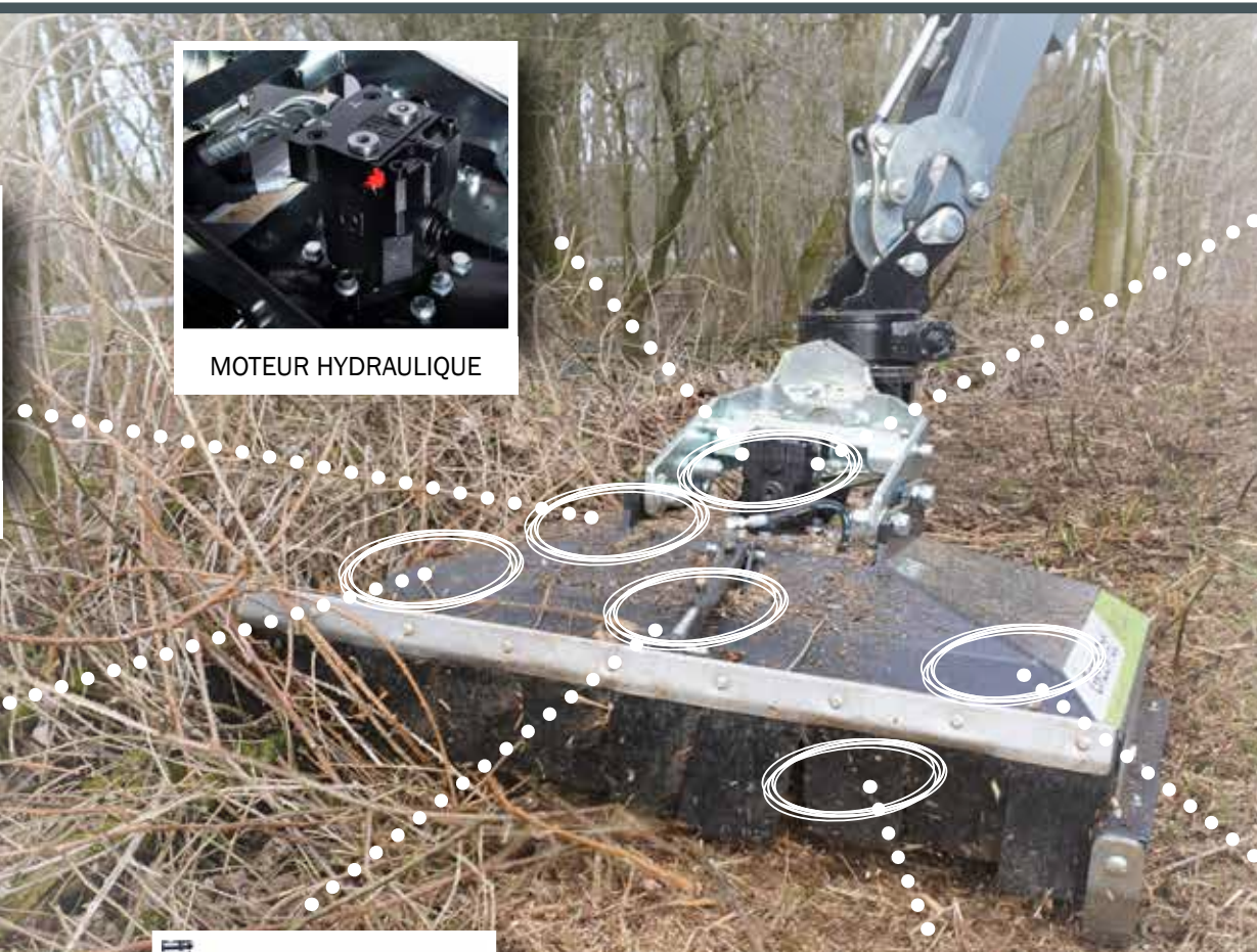
COUTEAUX OU CHÂÎNES
