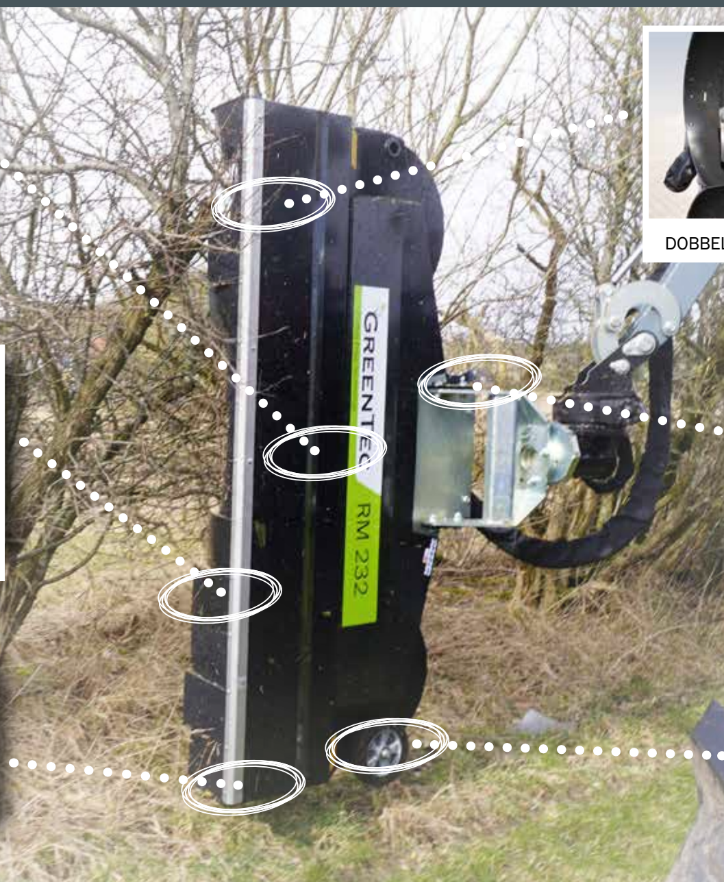
AFTAGELIG BUNDDÆKSEL
