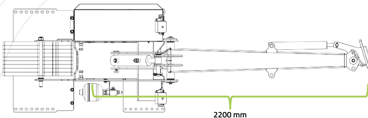
Figur 9 – Rækkevidde i arbejdsposition (fra midt-maskine u/ redskab): PUMA 2803 redskabsramme
