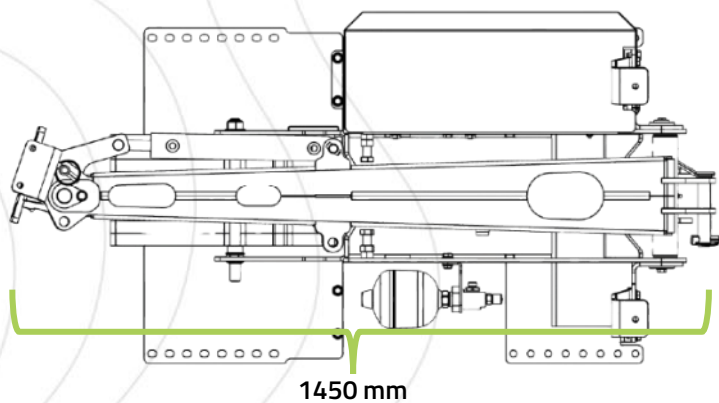
Figur 7 – Transportbredde (u/ arbejdsredskab): PUMA 2803 redskabsramme
