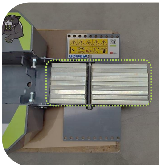
Kontravægte (85 kg.) monteret på PUMA 2803 redskabsramme
