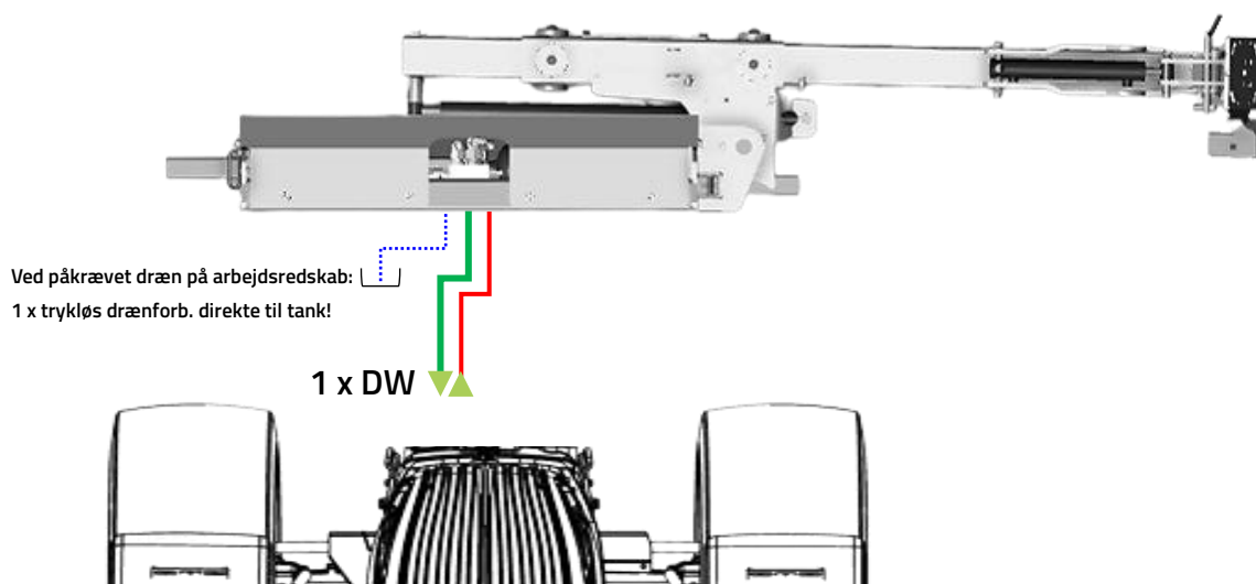
Hydrauliske slangeforbindelser mellem PUMA 2803 Tele redskabsramme og køretøj
