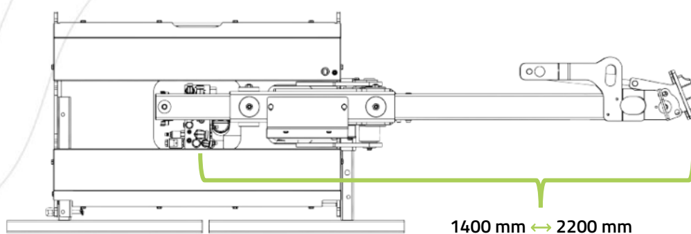
Figur 9 – Rækkevidde i arbejdsposition (fra midt-maskine u/ redskab): PUMA 2803 Tele redskabsramme
