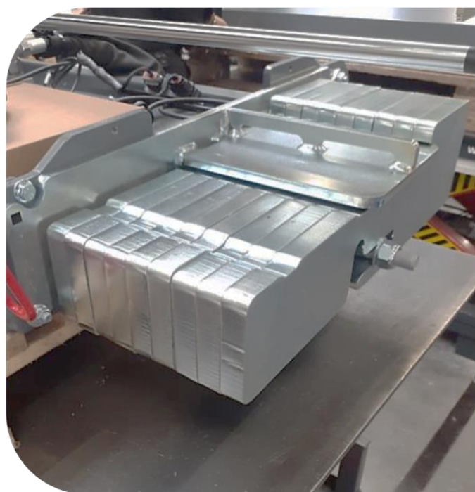
Kontravægte (85 kg.) på PUMA 2803 Tele redskabsramme
