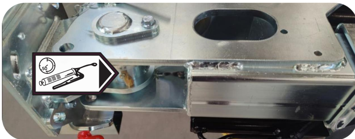
Placering af smørenippel yderst på PUMA 2803 Tele redskabsrammens teleskoparm
