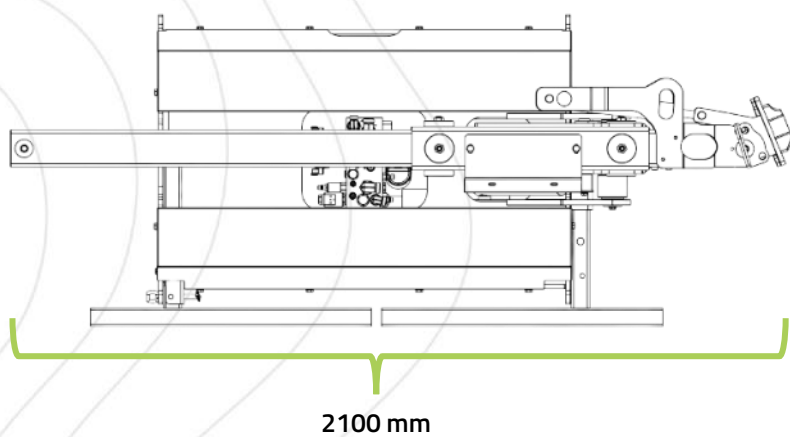
Figur 8 – Transportbredde (u/ arbejdsredskab): PUMA 2803 Tele redskabsramme
