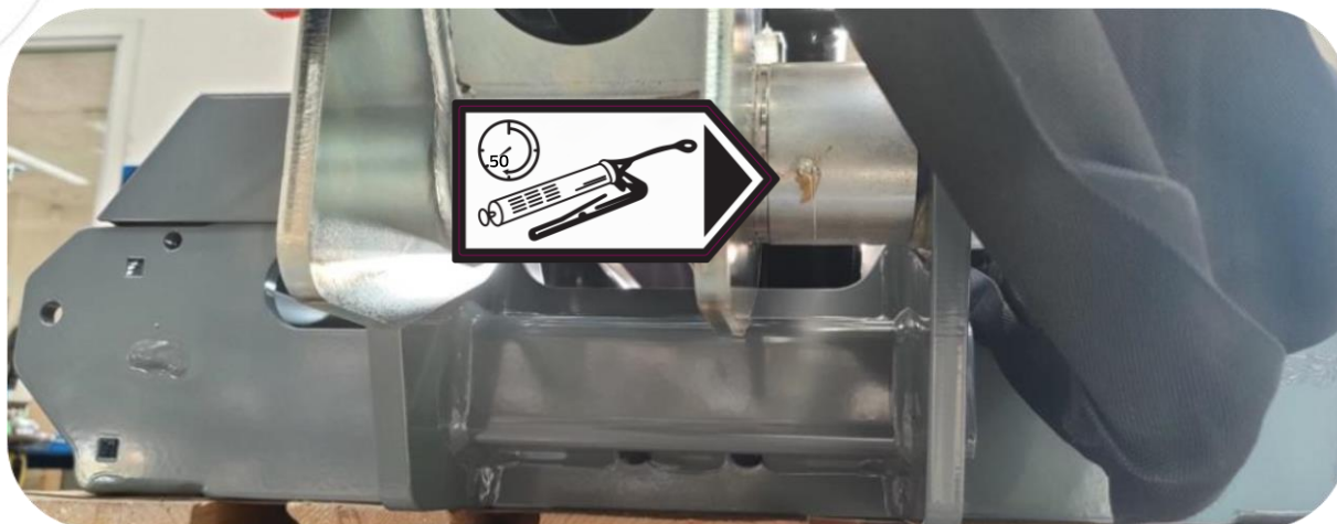
Placering af smørenippel inderst på PUMA 2803 Tele redskabsrammens teleskoparm
