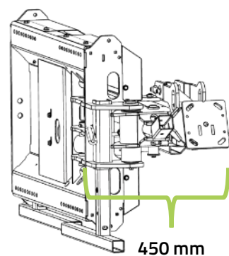
Figur 7 – Dybde (u/ læsserbeslag): PUMA 2803 Tele redskabsramme
