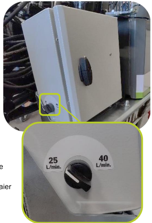
Schakelaar voor het veranderen van de olietoevoer naar het werktuig: 25 of 40
