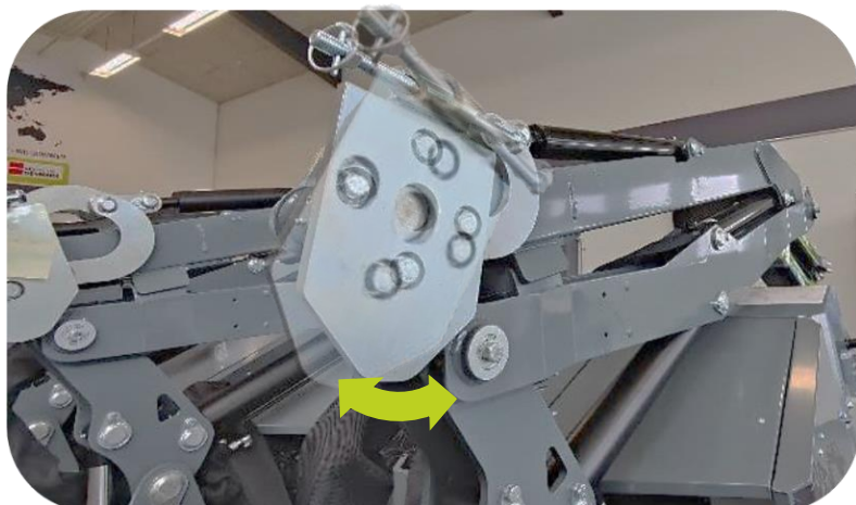
Mechanische snelkoppeling voor werktuigen op een Scorpion 3-430 Standaard
