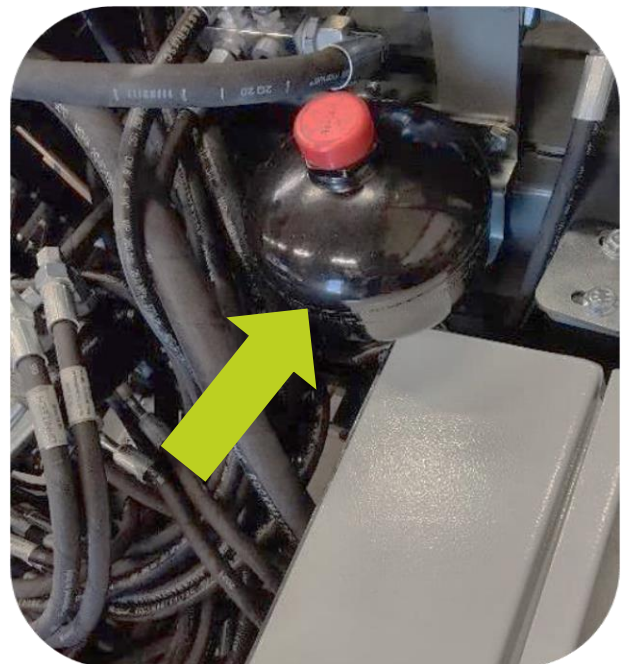
Accumulator (32 bar) op Scorpion 3-430 armmaaier
