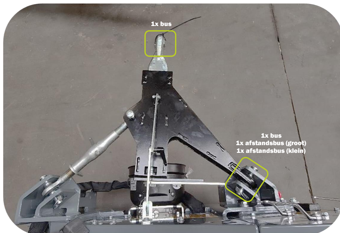
Bovenste trekstangen aangesloten op de montagebeugels van de Scorpion 3-430 armmaaier.
