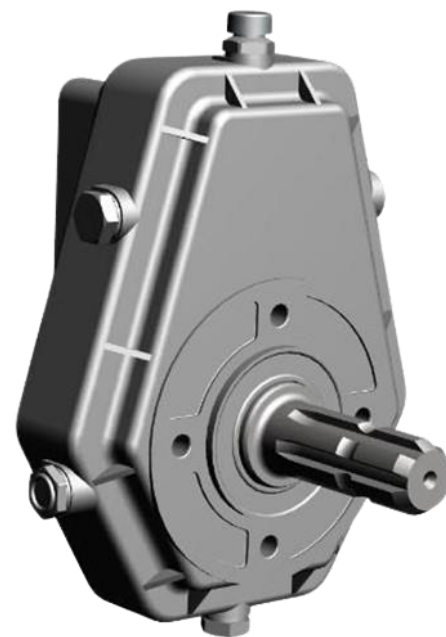
Versnellingsbak: Scorpion 3-430 armmaaier
