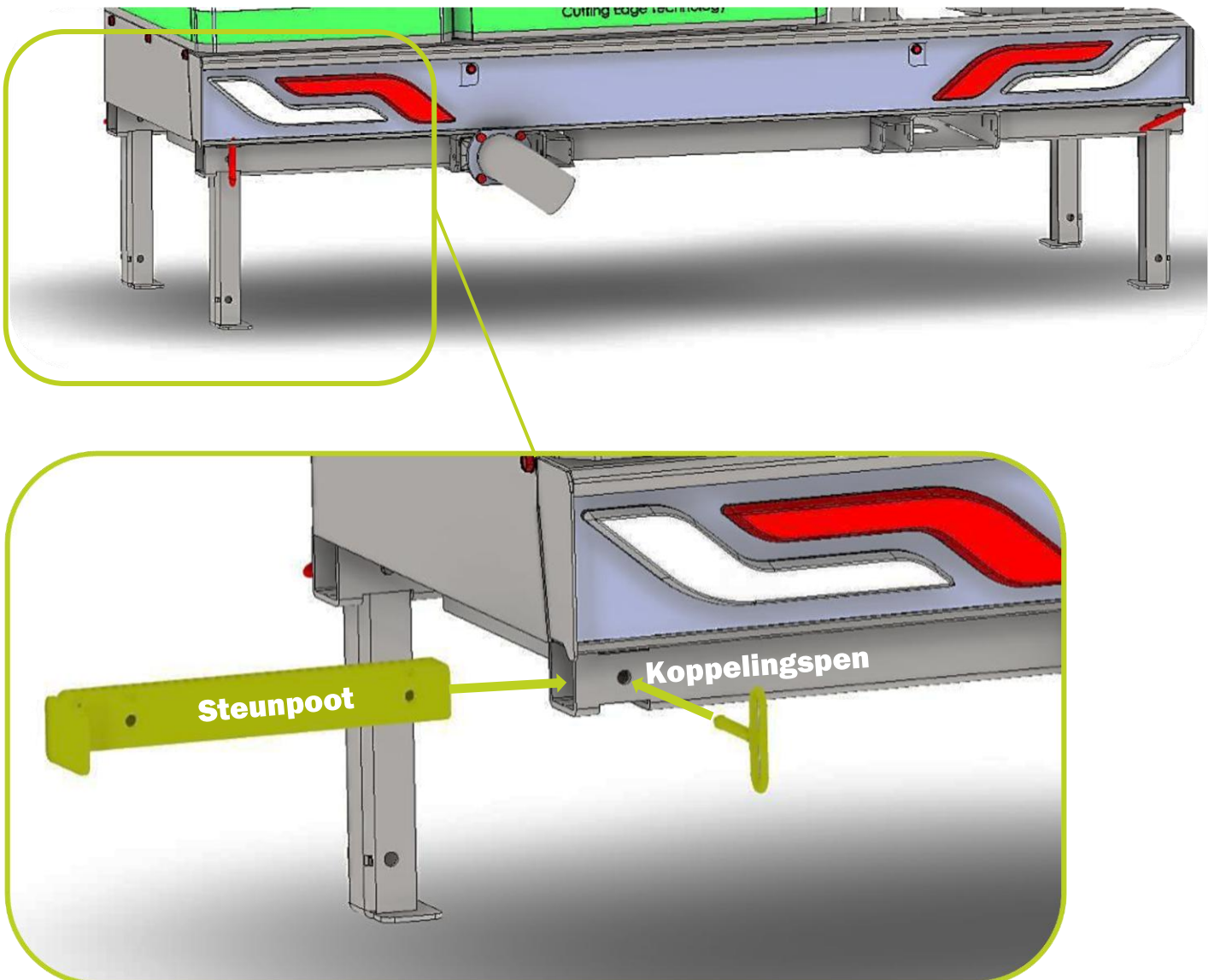
De locatie en werking van de steunbokken
