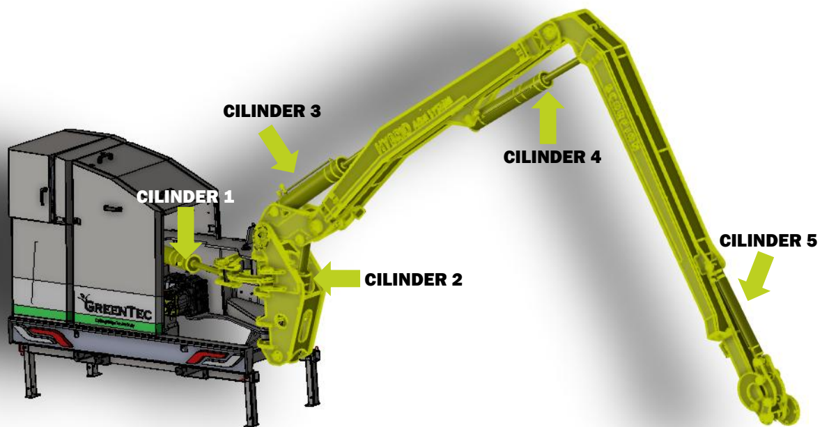
Overzicht: hydraulische cilinder op Scorpion 5-830 armmaaier
