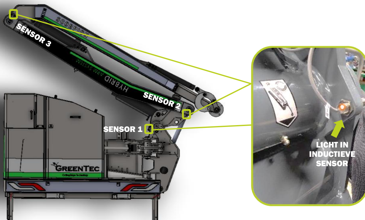
Locatie van inductieve veiligheidssensoren op Scorpion 5-830 armmaaier (3 stuks) - 1/2
