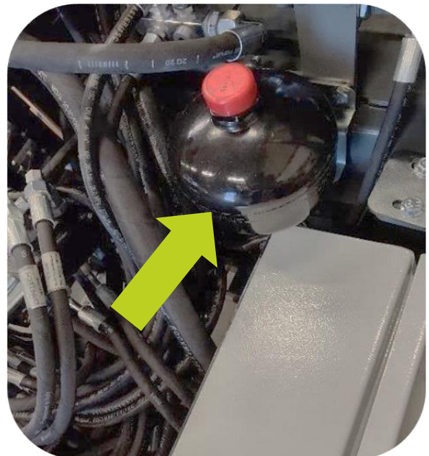
Accumulator (32 bar) op Scorpion 5-830 armmaaier
