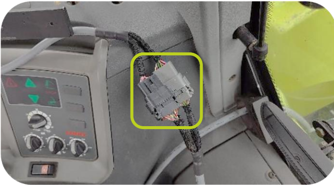
Het bedieningspaneel aansluiten met behulp van 2 stekkers/kabels van de armmaaiër naar de cabine van het voertuig
