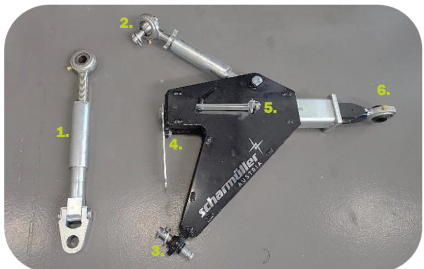
Onderdelen voor 4-punts hefinrichting systeem op Scorpion 5-830 armmaaier
