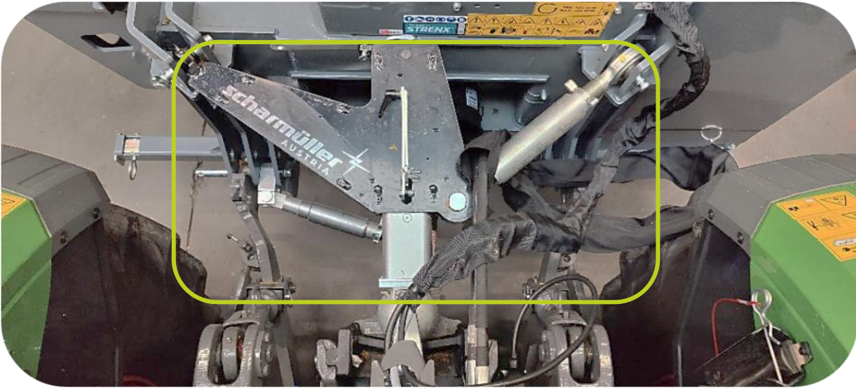
4-punts hefinrichting systeem: topstabilisatie op Scorpion 5-830 armmaaier
