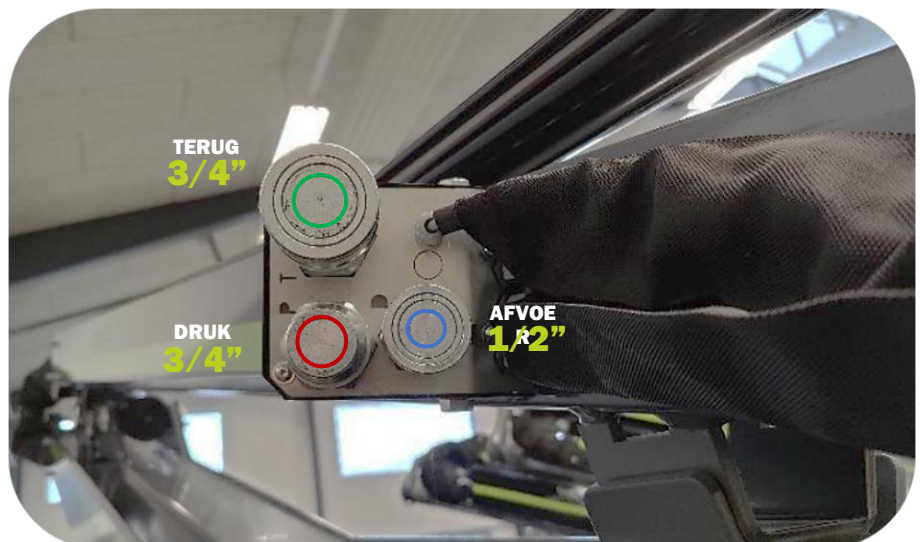
Aansluitingen/uitgangen voor hydraulische snelkoppelingen aan de buitenkant van de hefarm van de
