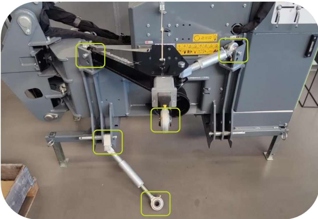
Plaatsing van onderdelen incl. busen en/of afstandsbusen in verband met 4-punts hefinrichting systeem
