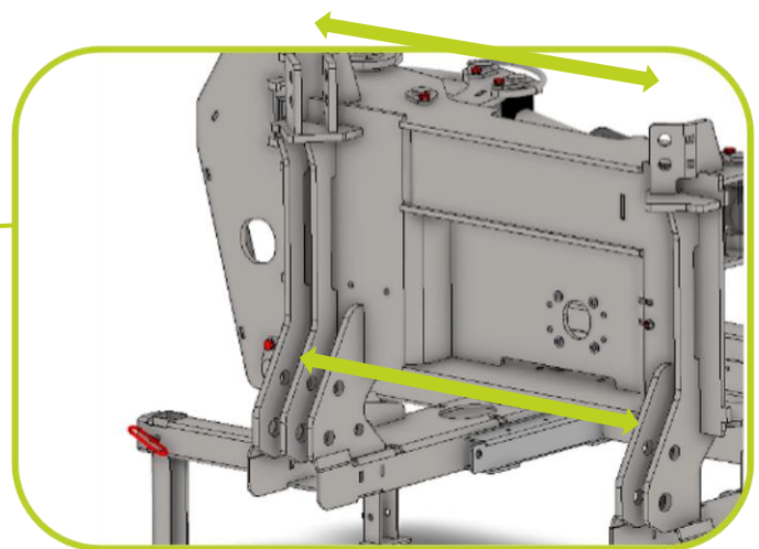
Beugels voor 4-punts hefinrichting: Cat. 1, 2 of 3
