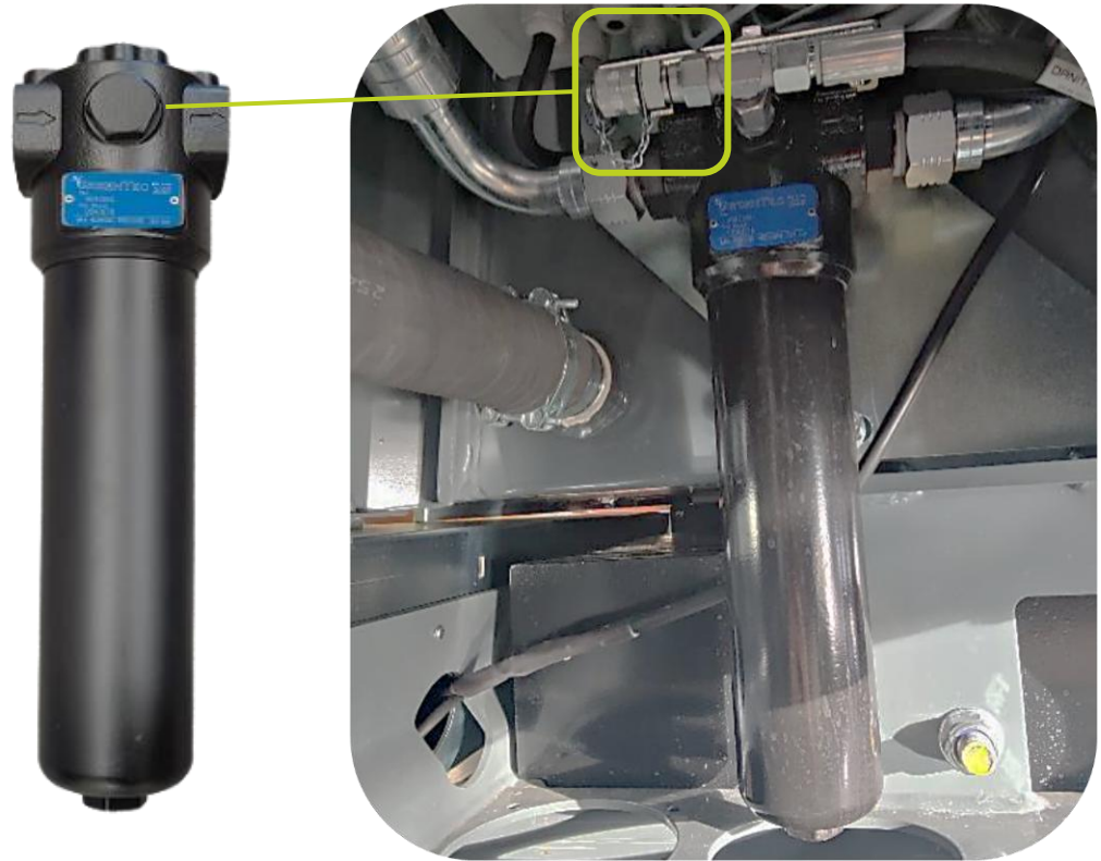
Uitgang/aansluiting voor manometer op het hogedrukfilter
