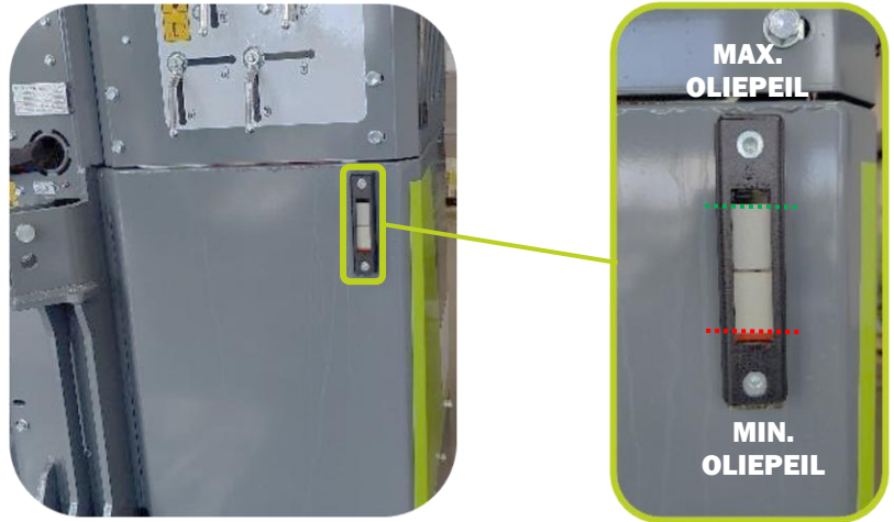
Plaats van de oliepeilmeter op de Scorpion 5-830 armmaaier
