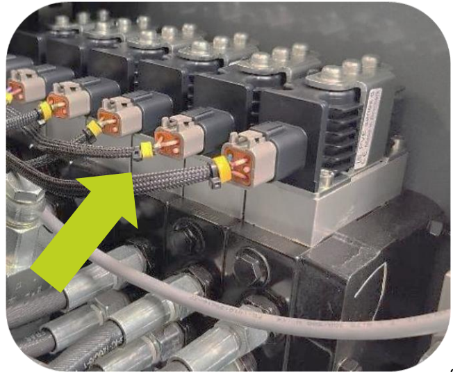
Danfoss PVG klep op Scorpion 5-830 armmaaier
