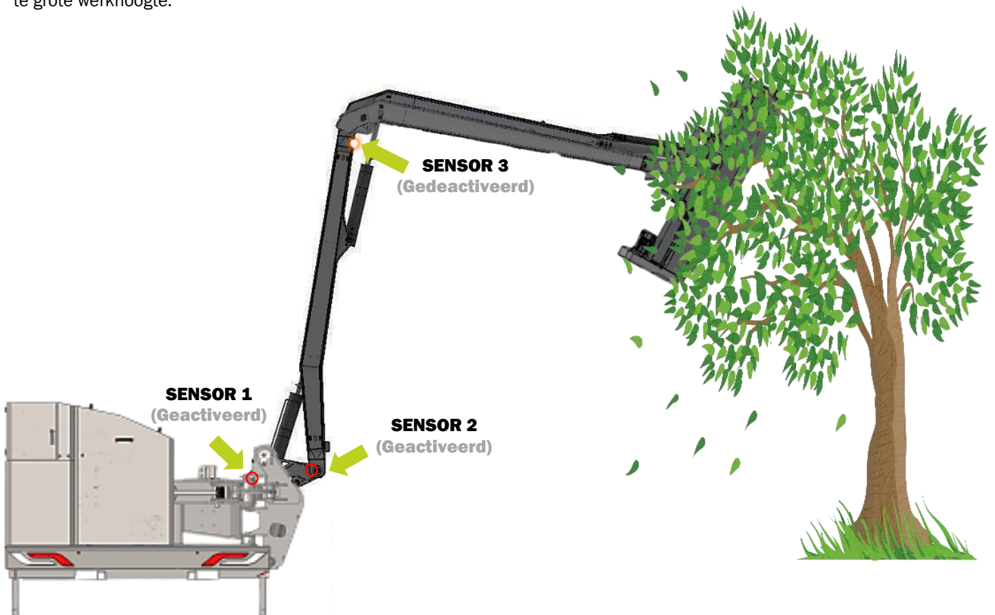
Veiligheidssensoren met arm gedeeltelijk uitgeschoven: Scorpion 5-830 armmaaier
