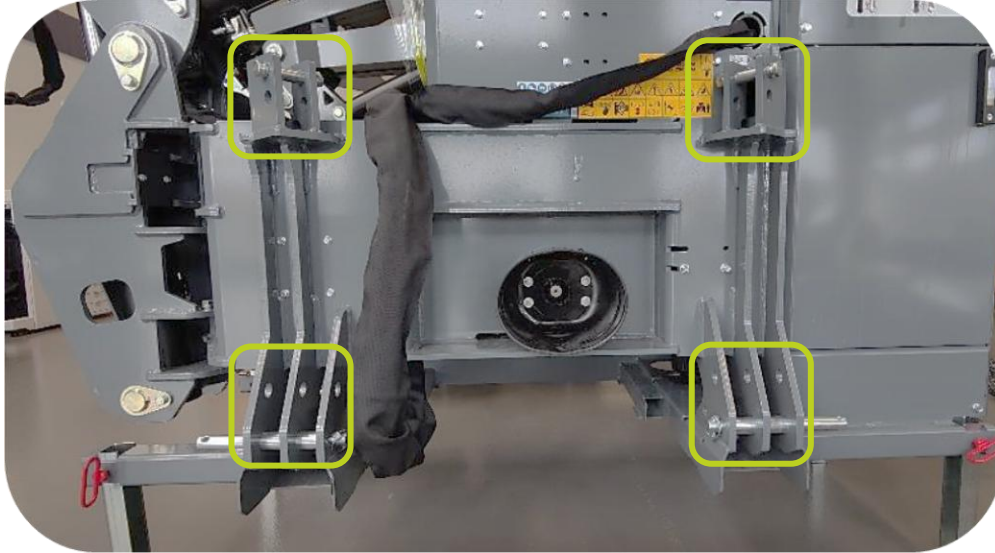
Montagepunten op Scorpion 5-830 armmaaier (cat. 2, 3 of 4)
