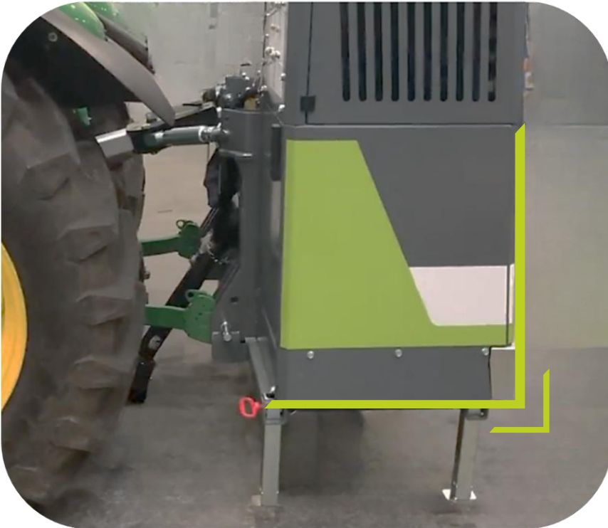
Scorpion 5-830 geheven door de hefarmen van het voertuig in verticale positie, na juiste instelling en
