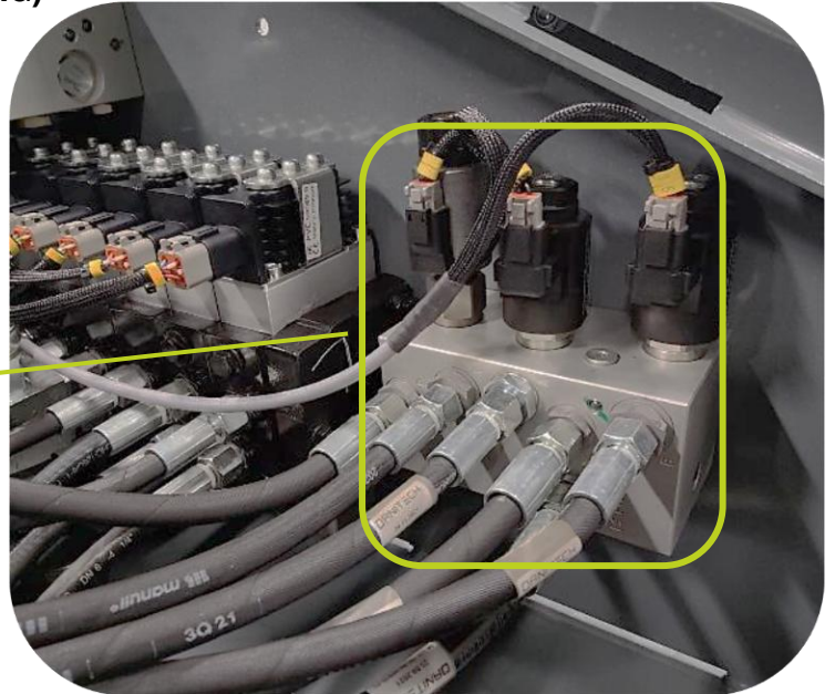
AHC-kleppenblok op Scorpion 5-830 armmaaier (optionele onderdelen)
