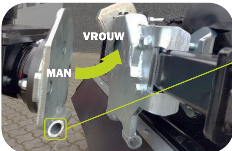
Mechanische snelkoppeling gemonteerd op Scorpion 5-830 Plus armmaaier met RotorFlex + "vrouwelijke" adapter gemonteerd op het hulpstuk
