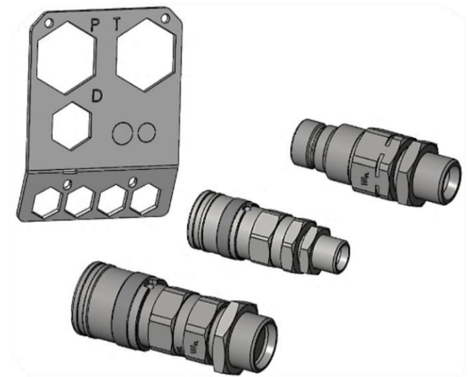
Vlakke snelkoppelingen voor de Scorpion 5-830 armmaaier
