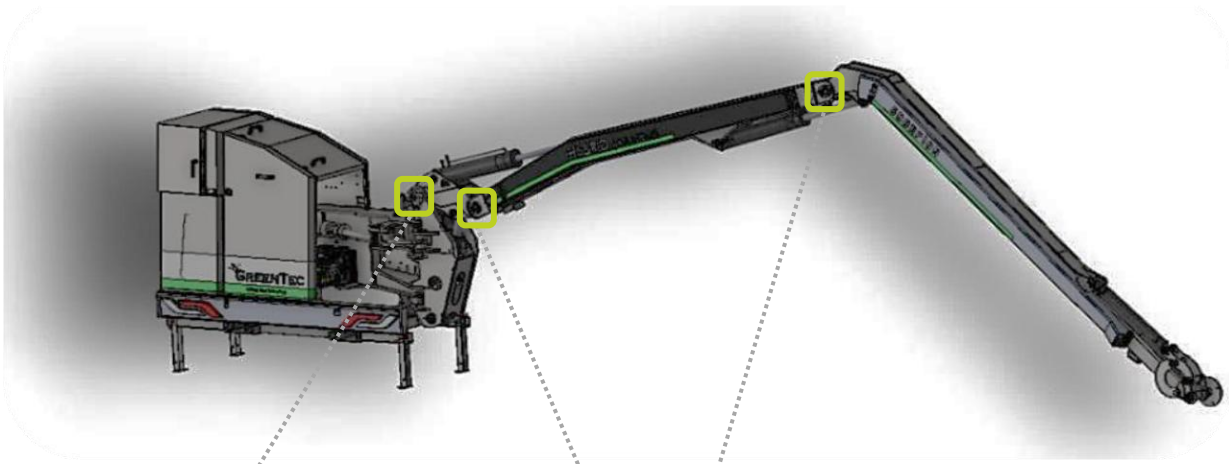
Plaats van inductieve veiligheidssensoren op Scorpion 5-830 armmaaier (3 stuks) - 2/2
