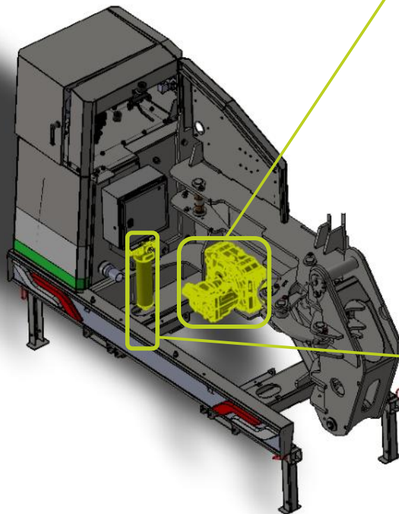
Locatie van versnellingsbak, hydraulische pomp en hogedrukfilter op Scorpion 5-830 armmaaier
