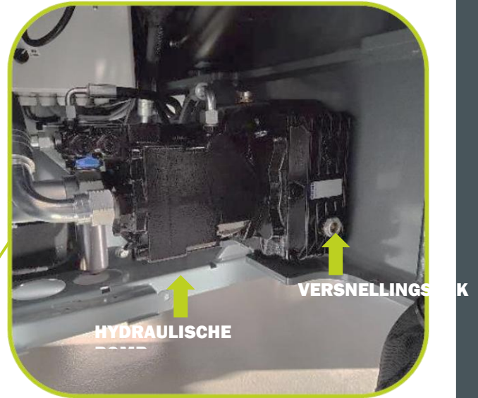
Hydraulische pomp en versnellingsbak (Zicht vanaf de onderkant van de Scorpion 5-830 armmaaier)
