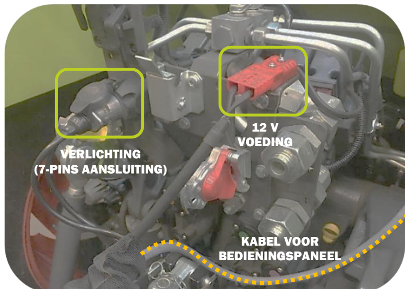
De Scorpion 5-830 armmaaier aansluiten op het voertuig
