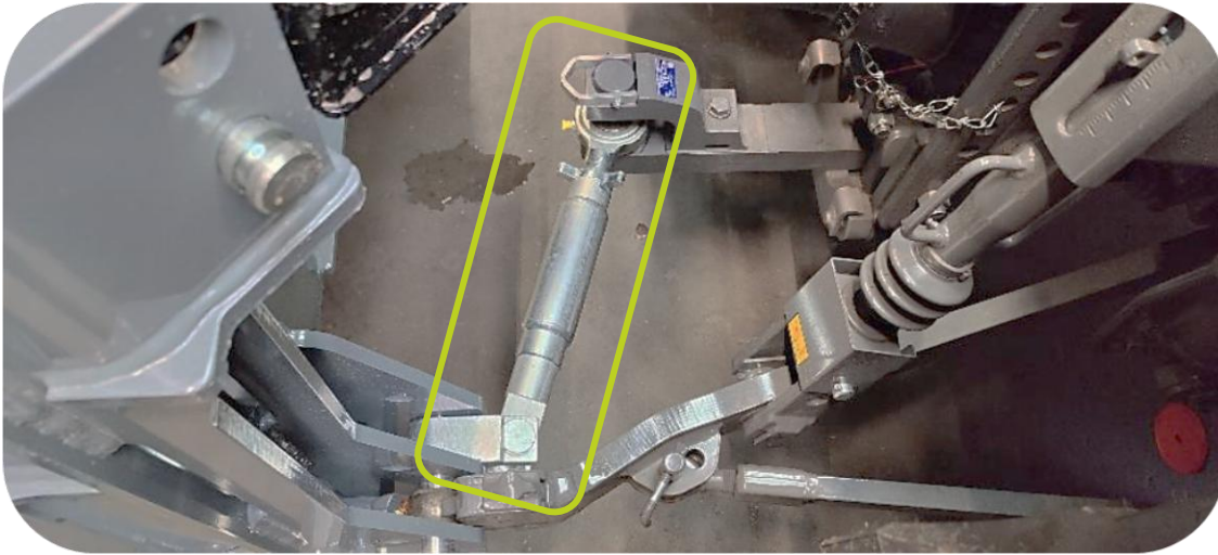
4-punts hefinrichting systeem: lagere stabilisatie op Scorpion 5-830 armmaaier
