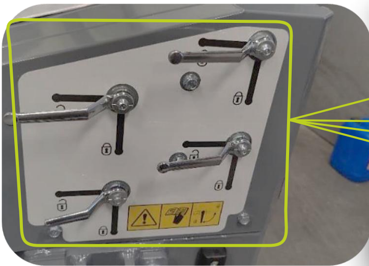
Stopkranen (4x) voor het blokkeren van cilinders tijdens transport en
