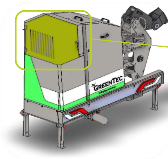
Plaats van retour oliefilter op de Scorpion 5-830 armmaaier
