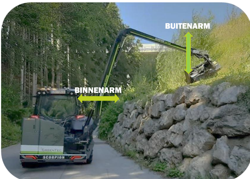
Scorpion 5-830 armmaaier in gebruik met niet parallelfunctie geactiveerd
