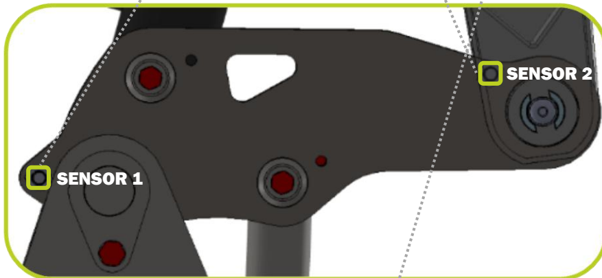
Plaats van inductieve veiligheidssensoren op Scorpion 5-830 armmaaier (3 stuks) - 2/2
