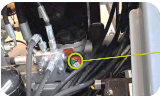
Manometer/indicator voor het vervangen van het
