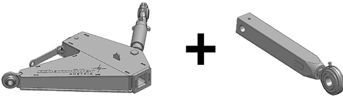
4-punts hefinrichting systeem: topstabilisatie op Scorpion 5-830 armmaaier
